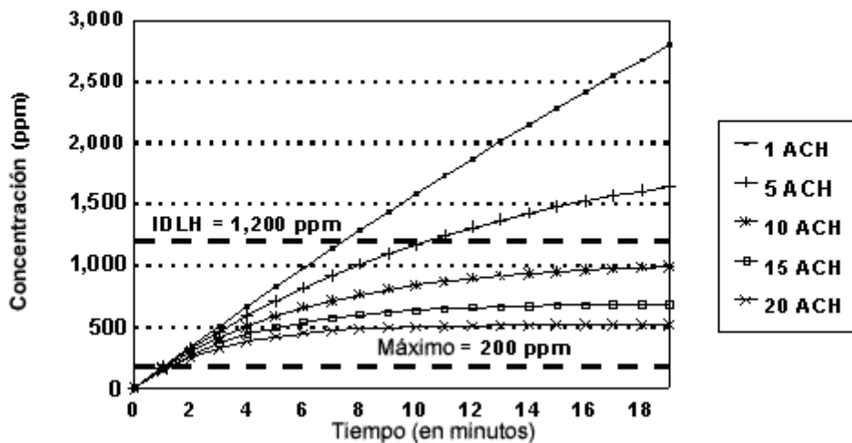
Figura 3. Concentraciones de CO calculadas que genera un motor de gasolina de 4 ciclos y 5 caballos de fuerza en un salón de 283 metros cúbicos (10,000 pies cúbicos) con varios cambios de aire por hora.
