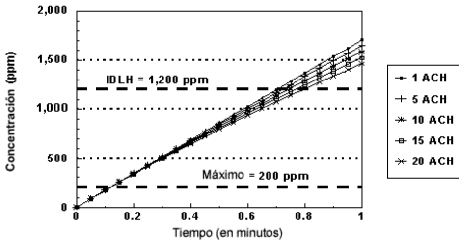
Figura 2. Concentraciones de CO calculadas que genera un motor de gasolina de 4 ciclos y 5 caballos de fuerza en un salón de 283 metros cúbicos (1.000 pies cúbicos) con varios cambios de aire por hora.
