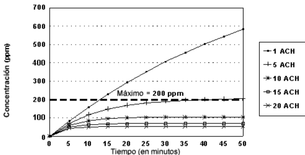
Figura 4. Concentraciones de CO calculadas que genera un motor de gasolina de 4 ciclos y 5 caballos de fuerza en un salón de 283 metros cúbicos (100.000 pies cúbicos) con varios cambios de aire por hora.
